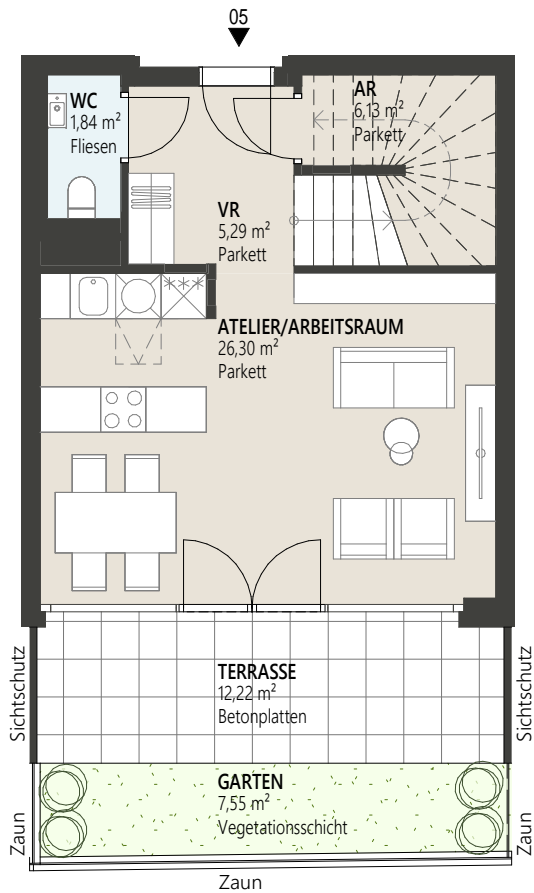
ERDGESCHOSS
