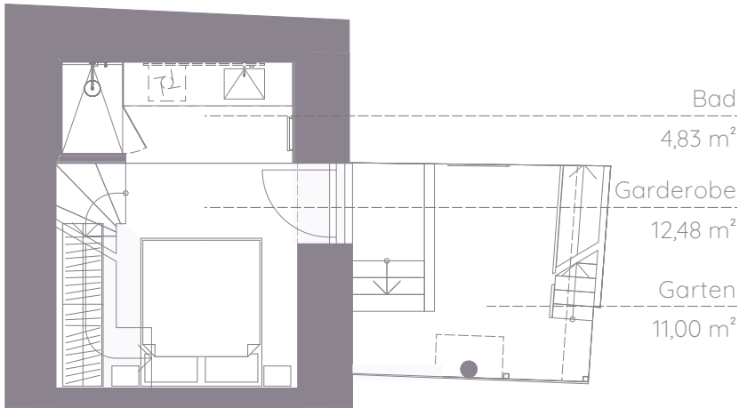
Gartengeschoß
